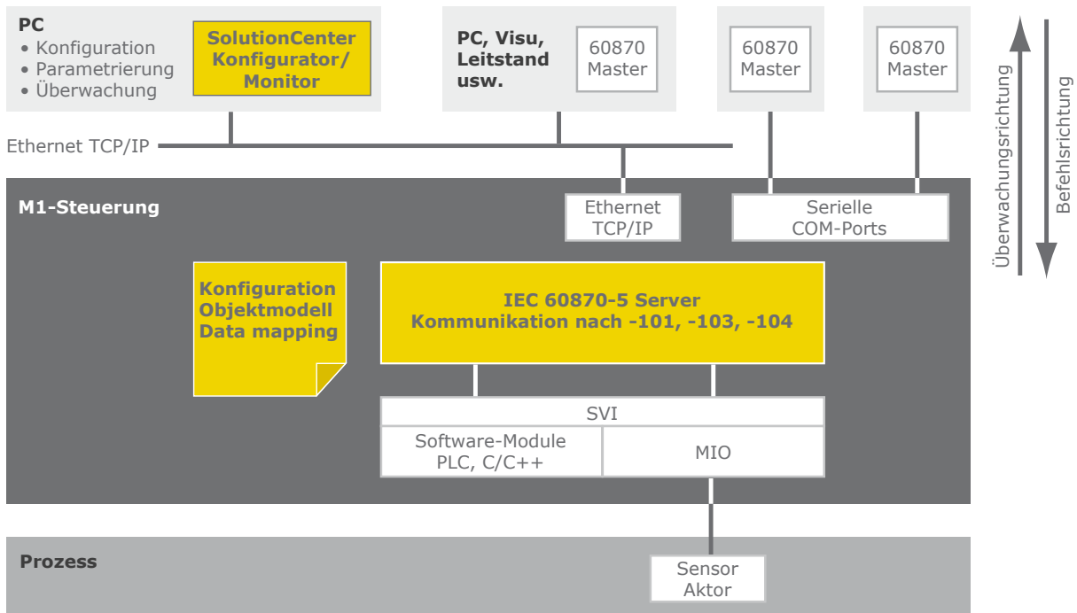
Blockschaltbild IEC 60870-5 Server
