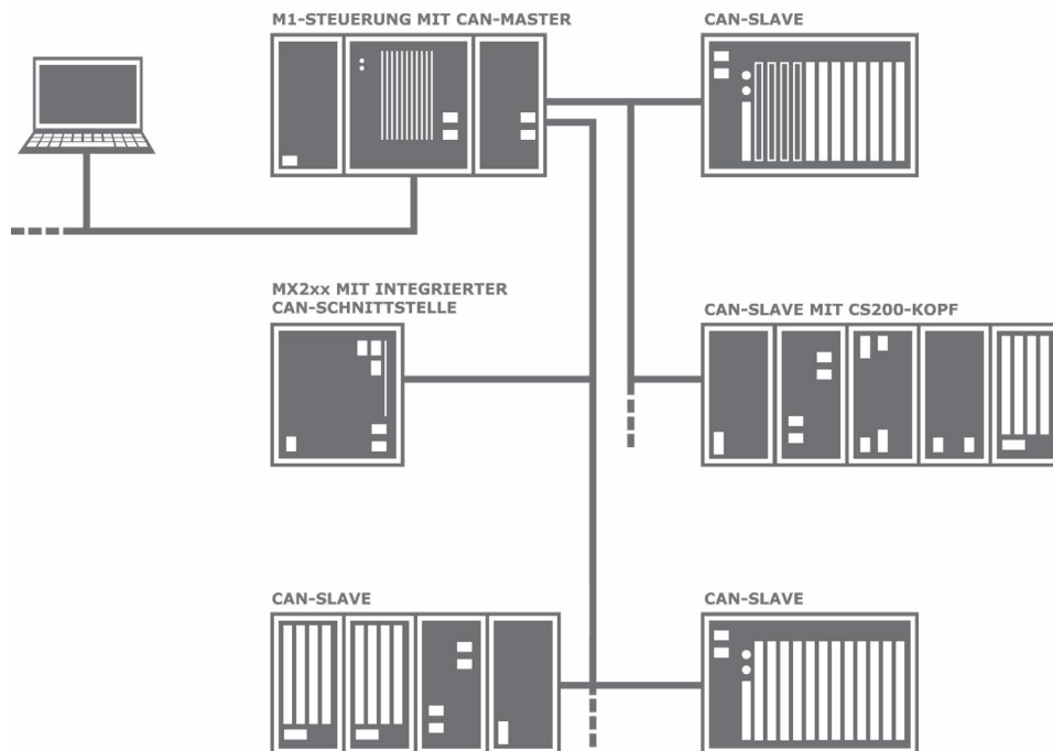
▶ Mögliche Topologie: CANopen
