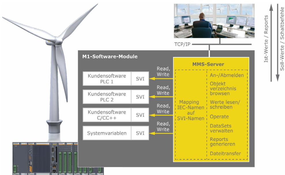
▼ MMS-Server als Scada-Schnittstelle zur M1-Steuerung
