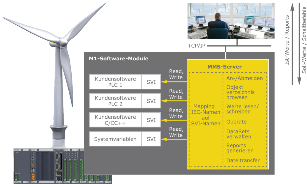
▼ MMS-Server als Scada-Schnittstelle zur M200-Steuerung
