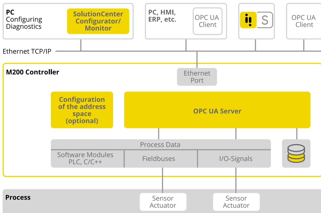
▼ OPC UA Server on the M200 controller
